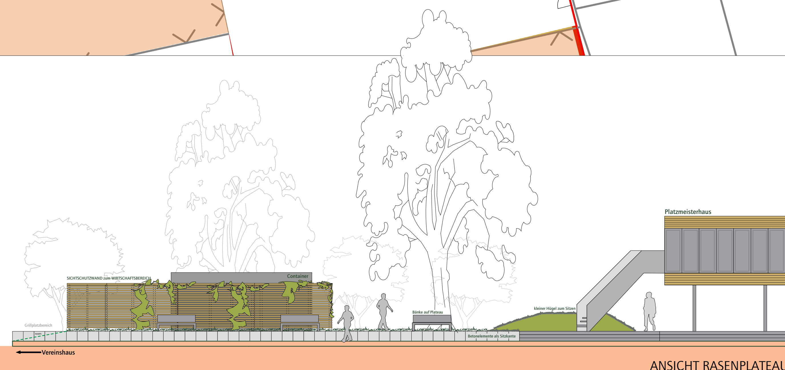
Auszug Freiflächenplan zu Umgestaltungsmaßnahmen/ Verfasser: (Vereinsmitglied) Yvonne Hirschmann_Architektin
